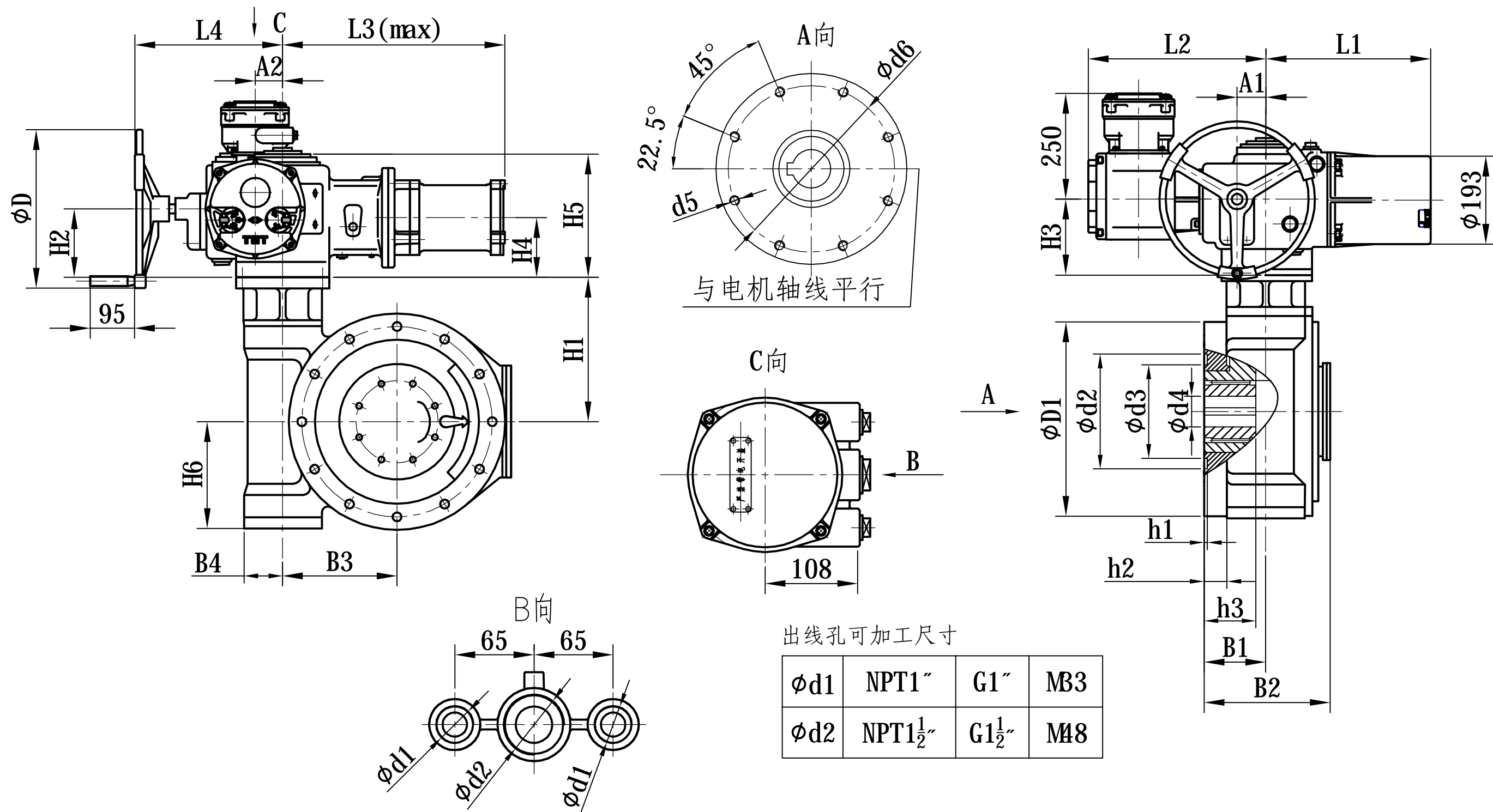
IMT-00 ~ 2/HBC 产品外型尺寸
