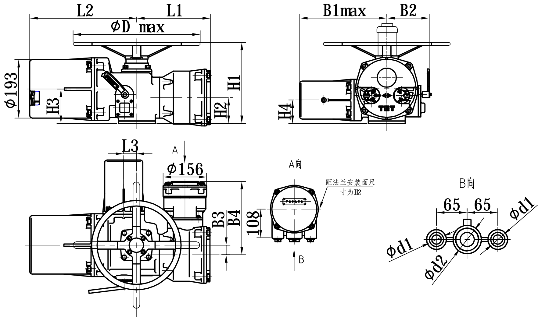
出线孔可加工尺寸
